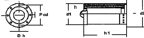
Typ DC mit Kalotte + 12 mm
